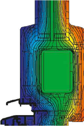
Tracé des isothermes Schüco LivIng AS porte d'entrée
