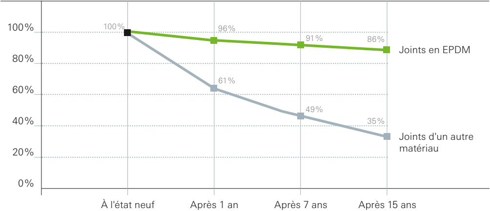
La technologie de joints habituelle forment des coins durs lors du soudage. Cela entraîne une perte d'élasticité et donc une étanchéité moindre.
